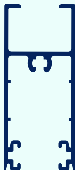
ZÓCALO Y CABEZAL DE HOJA (VS)
