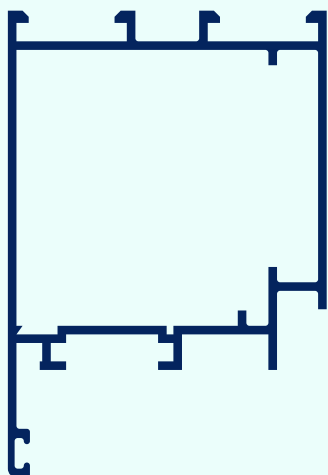
JAMBAL Y CABEZAL HOJA PUERTA DE REBATIR
